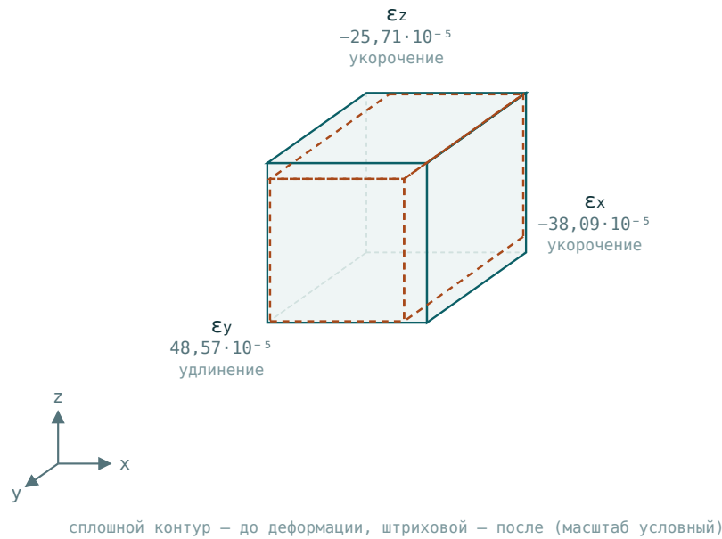
Рис. 1.4 — относительные линейные деформации: сплошной контур — до деформации, штриховой — после (масштаб условный).
