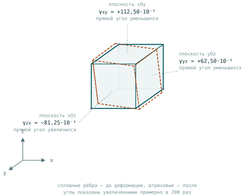
Рис. 1.5 — относительные угловые деформации на трёх координатных плоскостях. Сплошные рёбра — до деформации, штриховые — после; углы показаны увеличенными примерно в 200 раз (масштаб условный).
